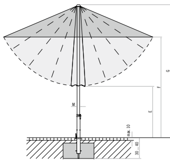
Betondicke 30 – 40 cm (Frosttiefe beachten), davon loser Deckbelag max. 10 cm, Wasserabfluss.
